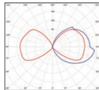
Modèle 1 E27 (2450 lm) Flux sortant - 1180 lm
