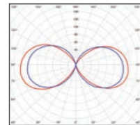
Modèles 2, 3 E27 (2450 lm) Flux sortant - 2100 lm
